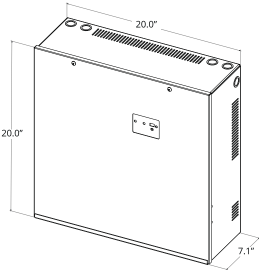
E3MINI 375VA
