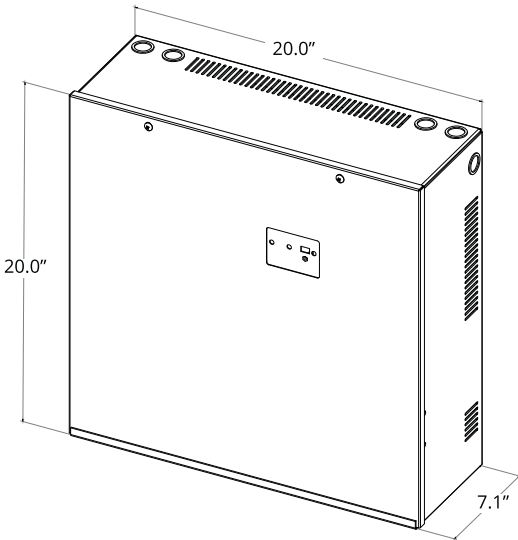
E3MINI 550VA
